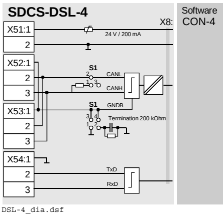
DSL-4_dia.dsf
