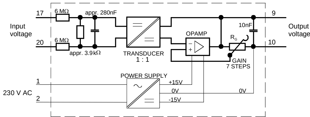
DC-DC 变换器 A92 的原理图
