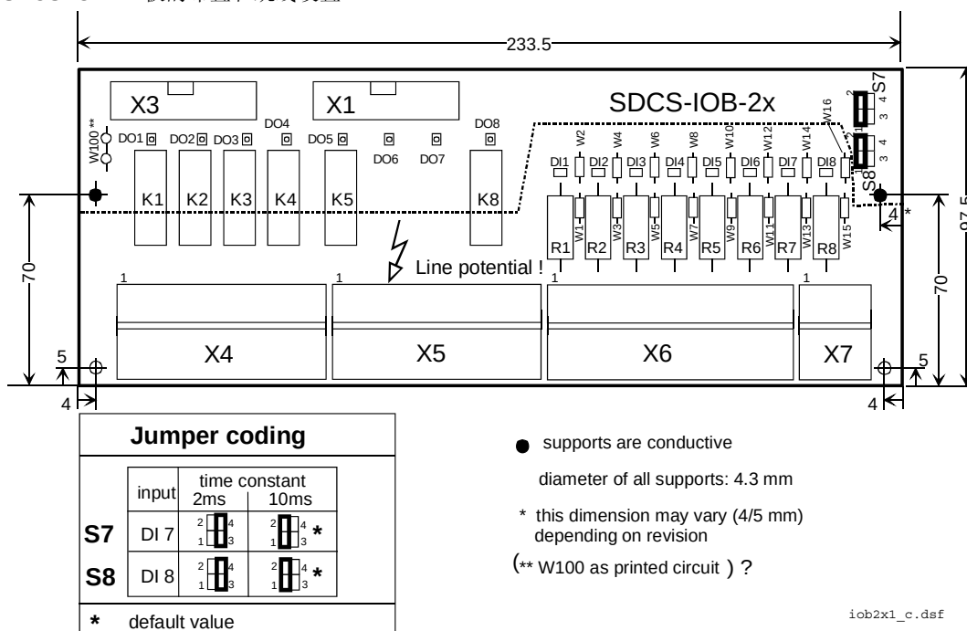
SDCS-IOB-2x 板的布置和跳线设置
