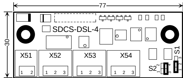
DSL-4_drw.dsf
