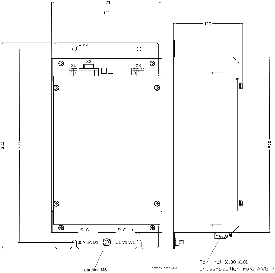
尺寸图
