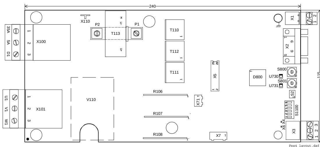
SDCS-FEX-4 板的布局
