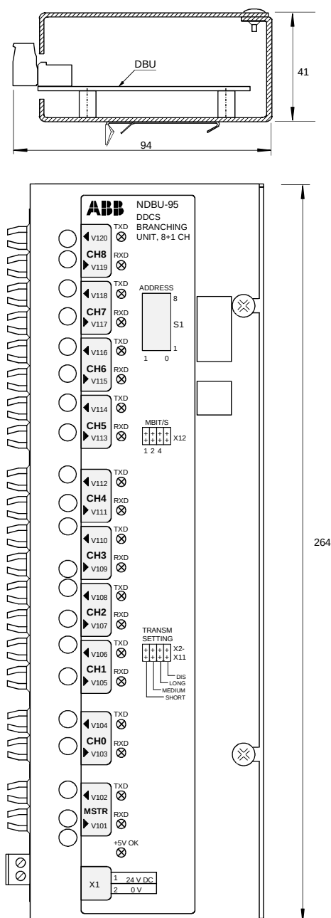
NDBU-95 分配单元外观图
