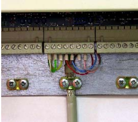
通过金属夹在变流器中 PCB 安装板的金属表面与电缆屏蔽层连接起来
