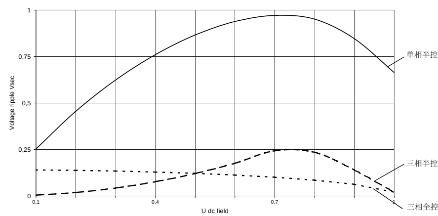
基于整流器工作模式的 U_{DC} 电压波动
