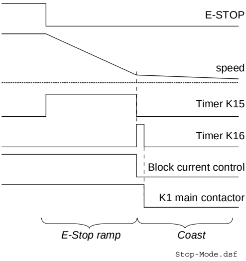
E-Stop 动作
